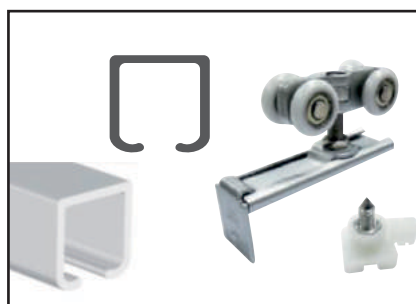
Item Code : DPS-047 80kg Specification : 1 Door kit
