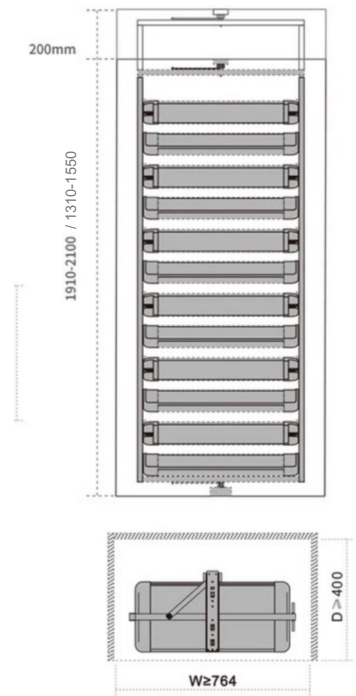
Shoe Rack Item Code : DPS-507 Pair Size : 8 shelf & 12 shelf Colour : Grey
